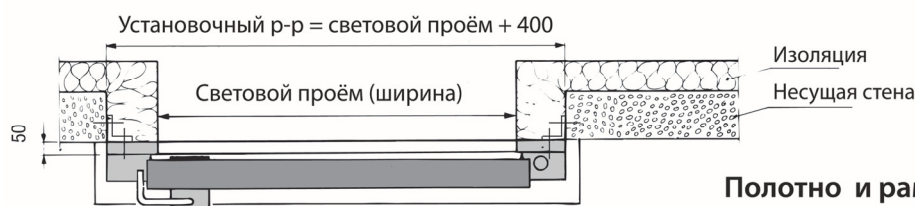
Показан вариант рамы (1)
