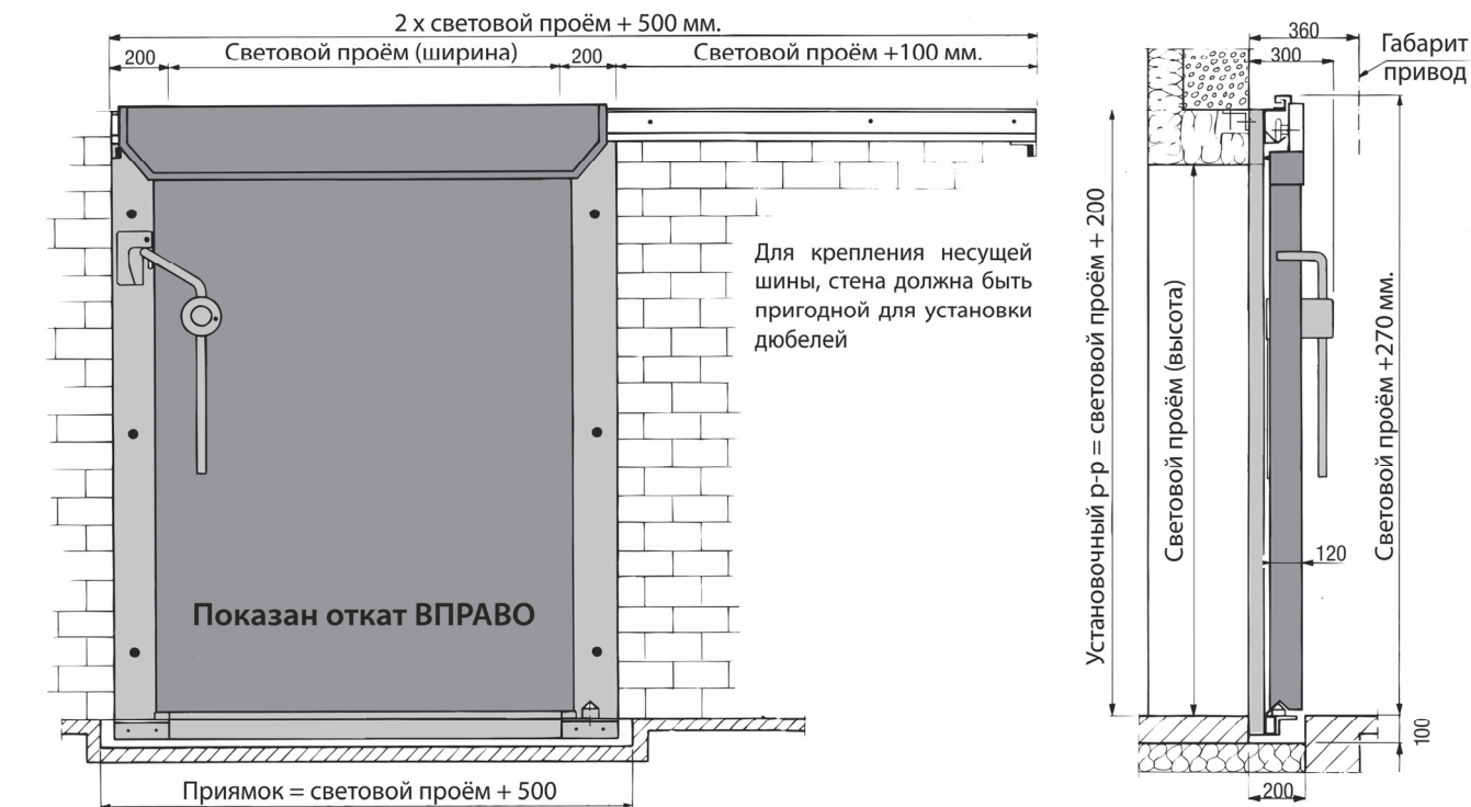
Показан вариант рамы (1)
